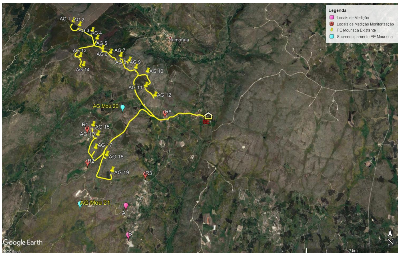
Figura 1: Representação dos locais de medição de ruído e localização do Sobreequipamento do Parque Eólico de Mourisca.
